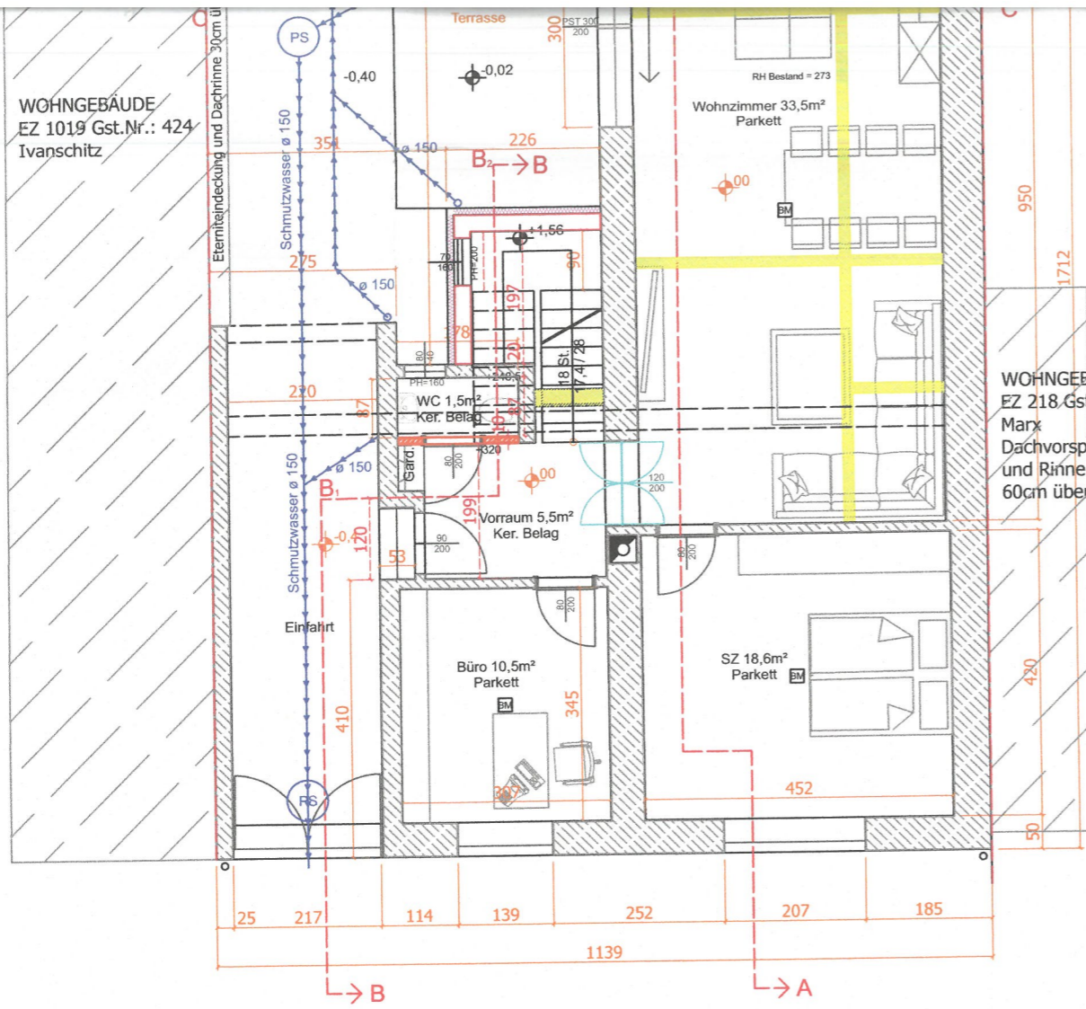
GRUNDRISS EG
