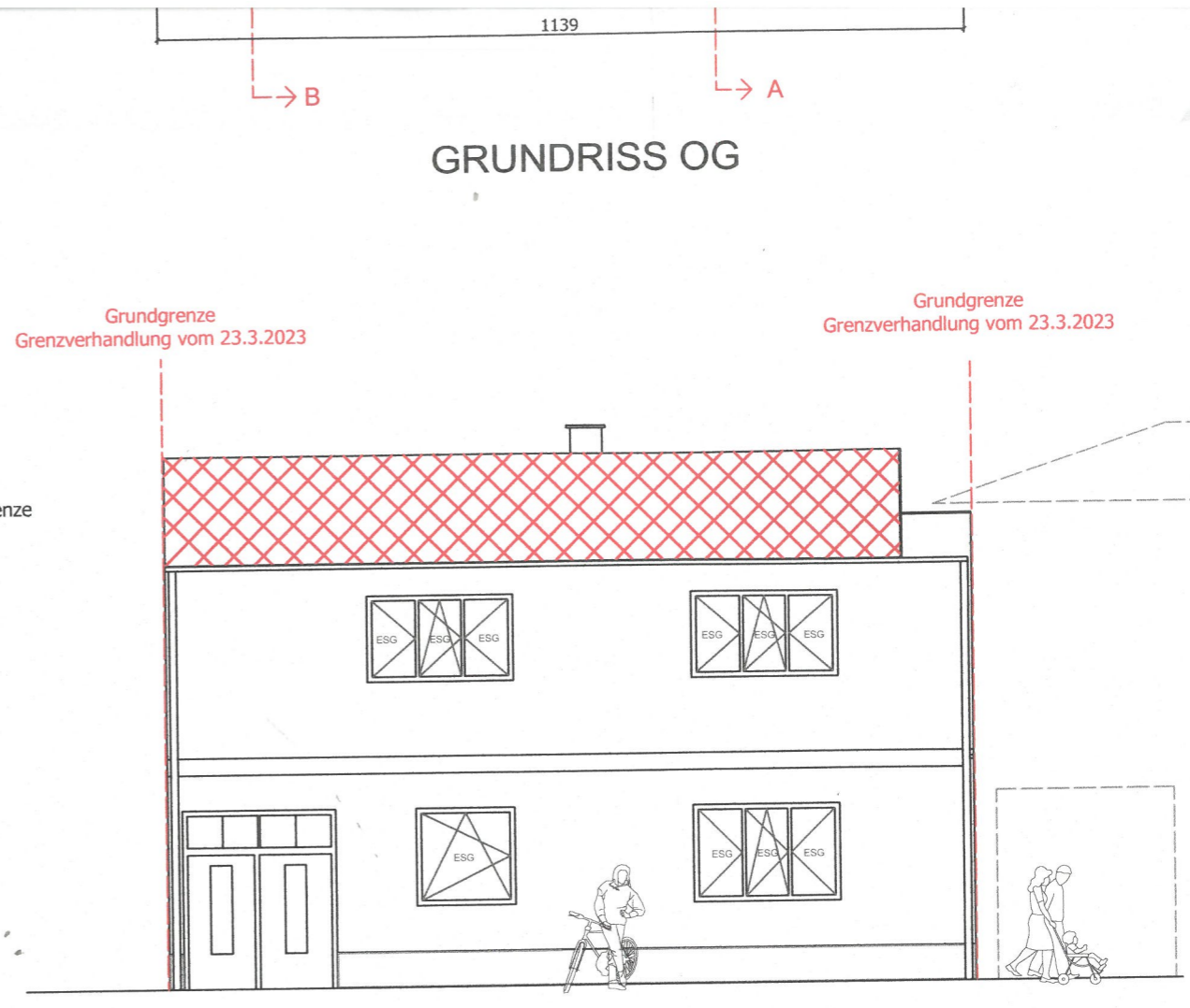
ANSICHT STRASSE
