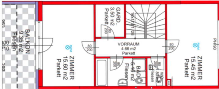
2. Obergeschoß Plan
