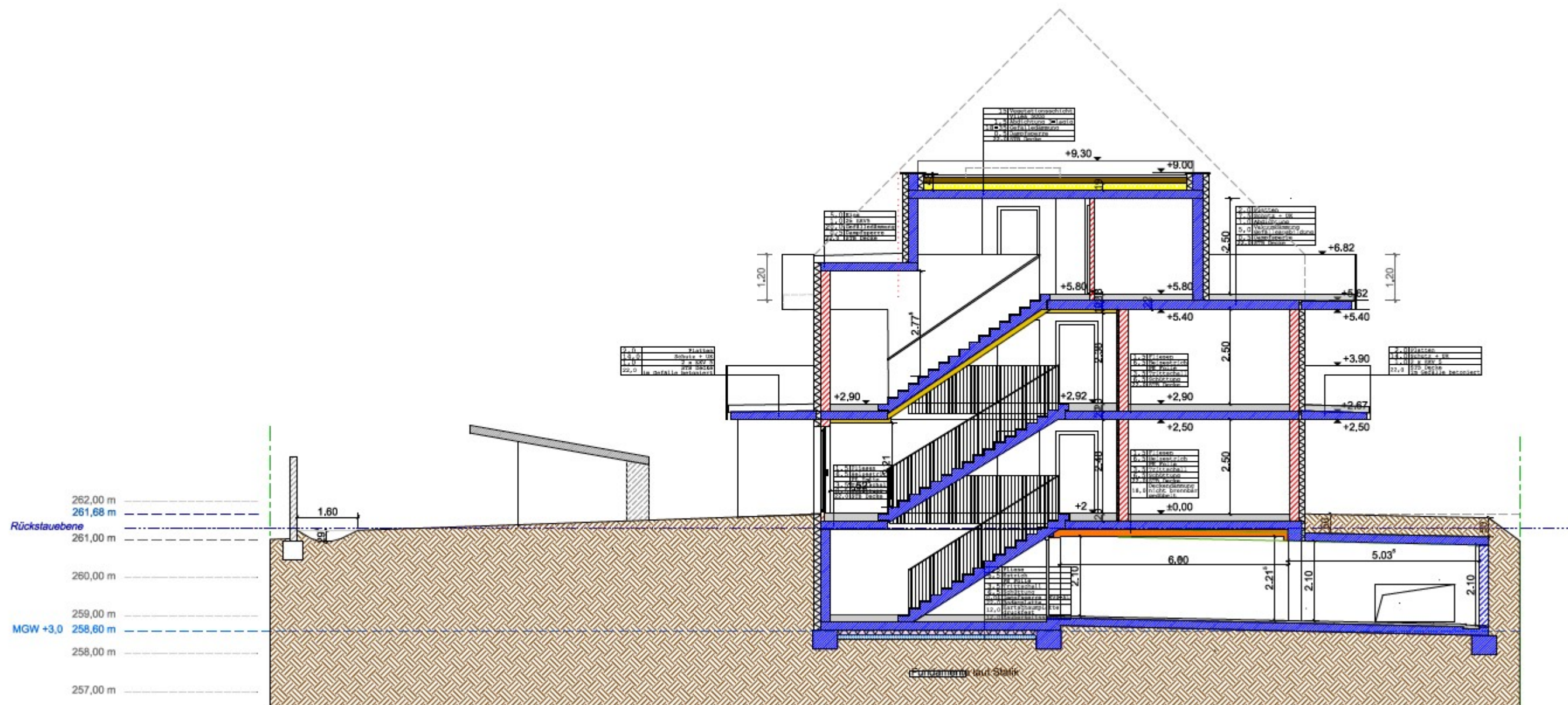
SCHNITT A-A M 1:100 138/37
