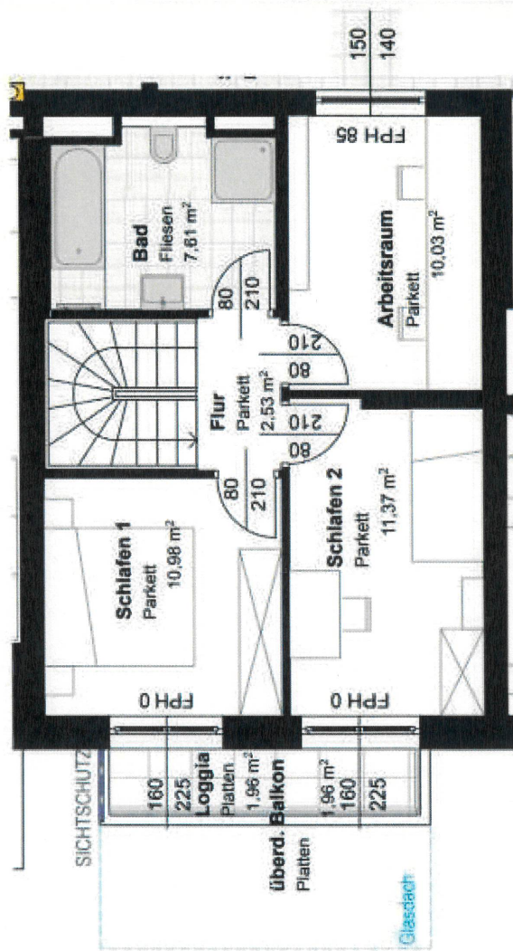
Grundriss 1. OG
