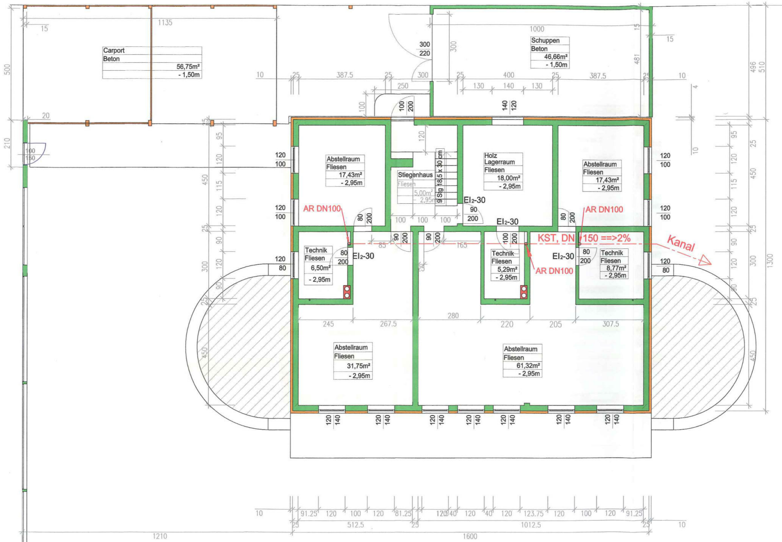
Schnitt Keller M1:100
