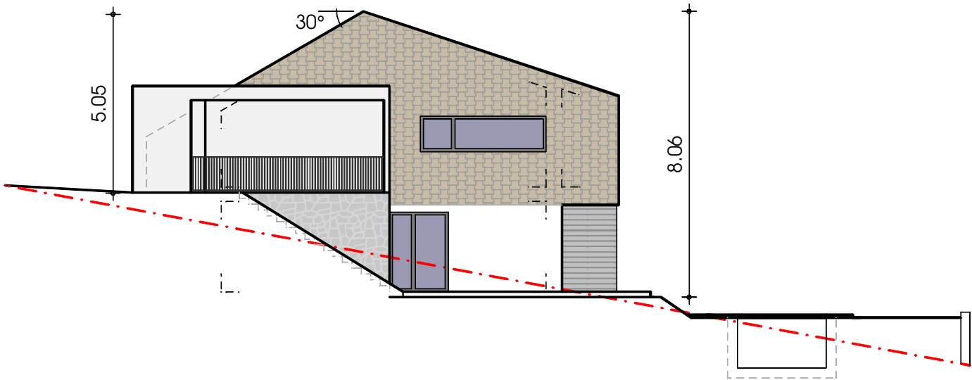
ANSICHT WEST
