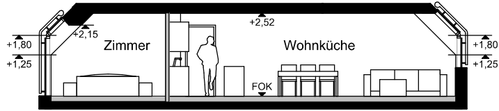
Querschnitt M:1:150 Wohnküche und Zimmer
