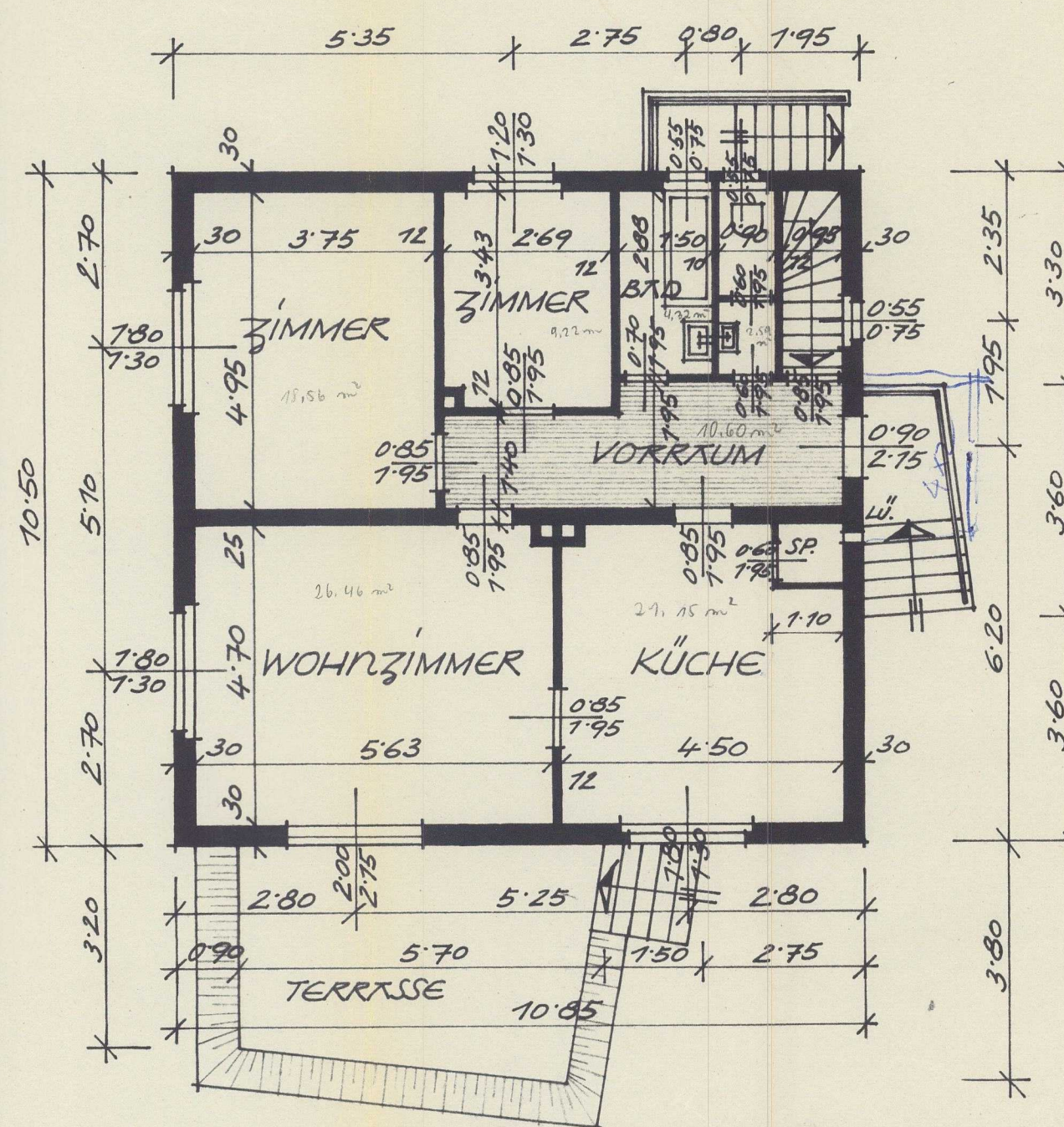
ERDGESCHOß
