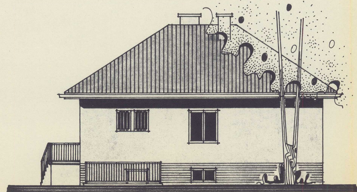
NO-ANSICHT
