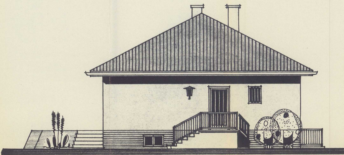
SO-ANSICHT
