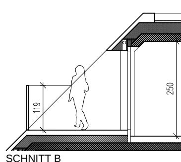
SCHNITT B
