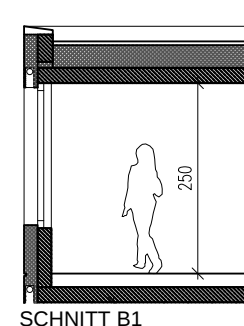
SCHNITT B1
