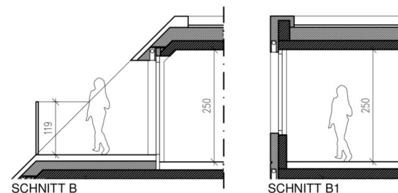
SCHNITT B
