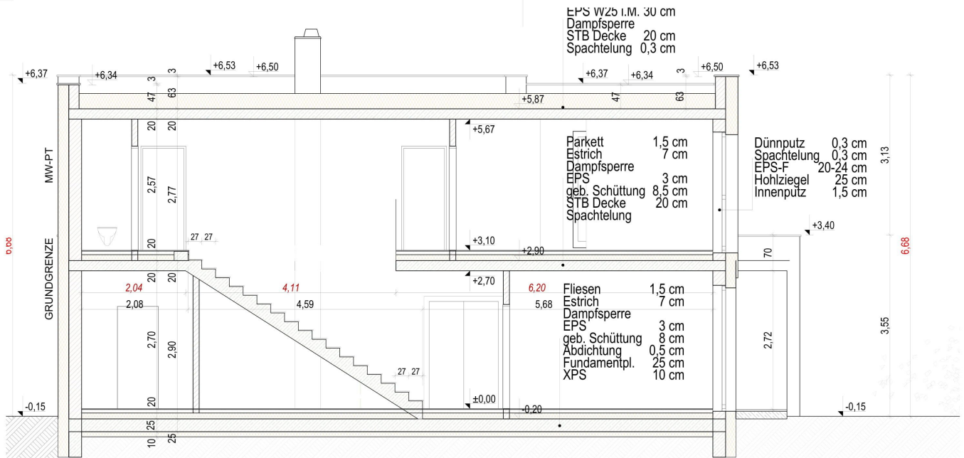
SCHNITT 1
