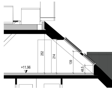
Schnitt 20.C
