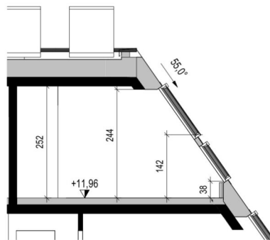
Schnitt 20.B
