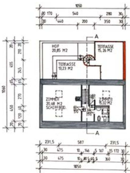
DACHGESCHOSS M 1:100
