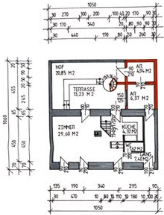
ERDGESCHOSS M 1:100
