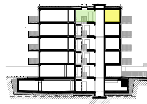
Schema Querschnitt
