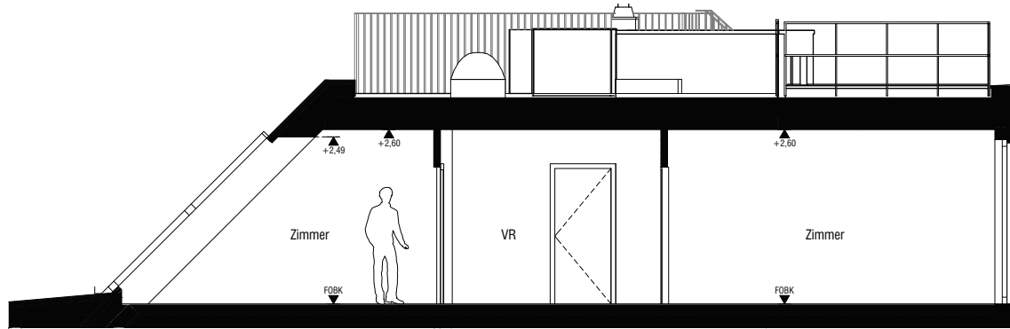
Schnitt
