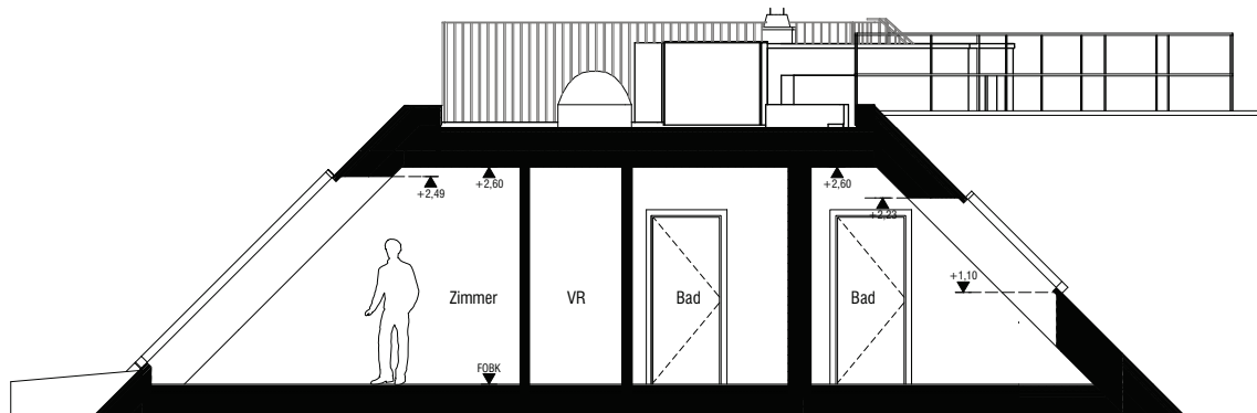
Schnitt
