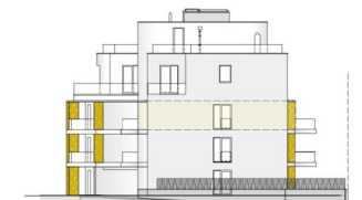
FASSADENANSICHT
