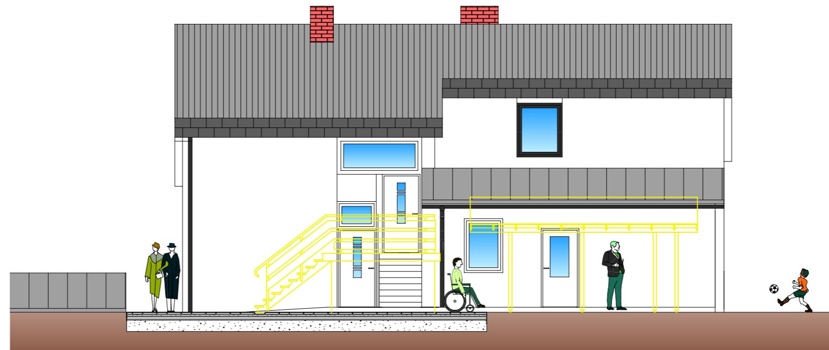
NORDANSICHT
