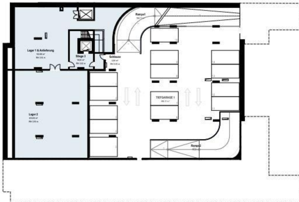
UNTERGESCHOSS
