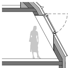
SCHNITT A
