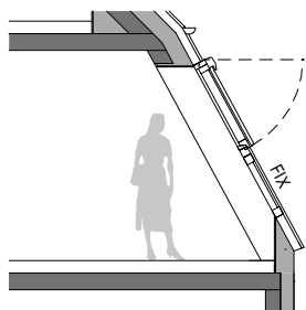
SCHNITT B
