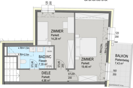
Grundriss DG:
