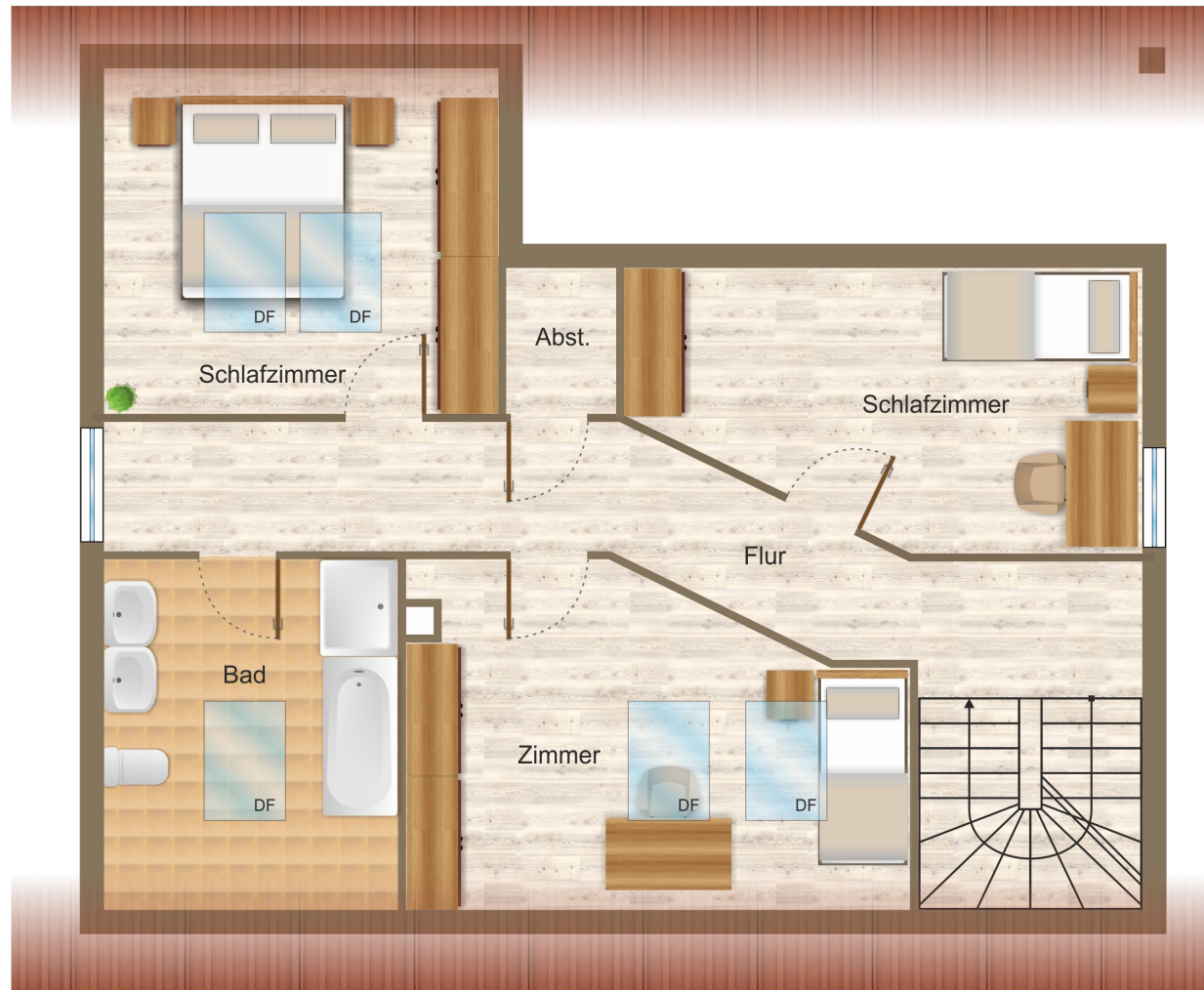
1. Obergeschoss
