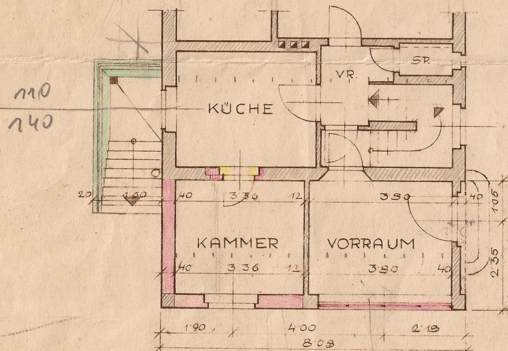
ERDGESCHOSS
