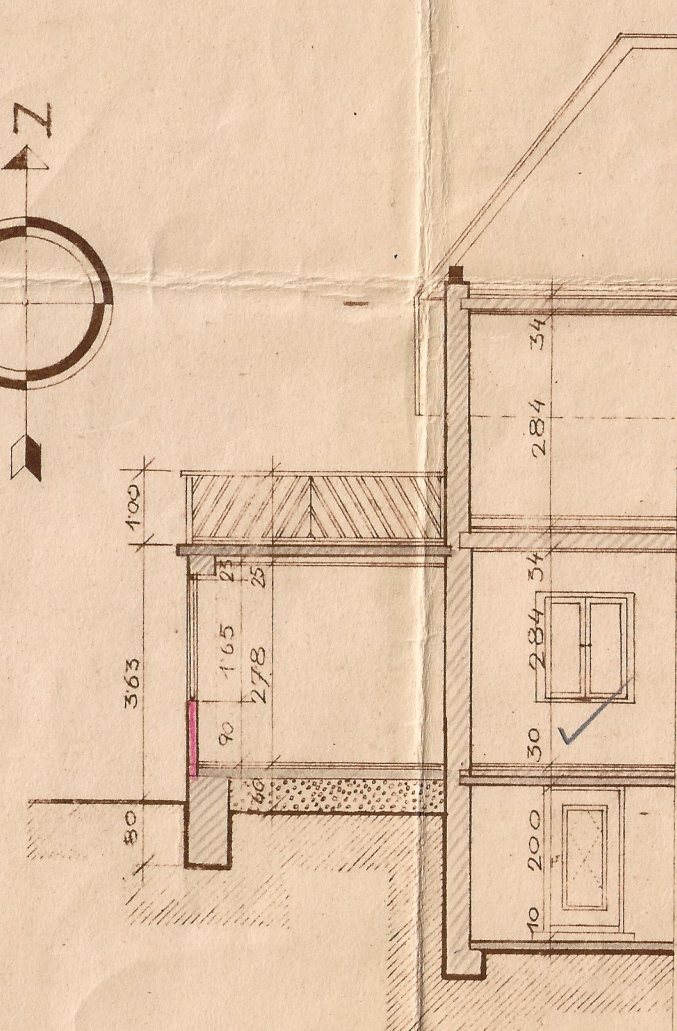
SCHNITT
