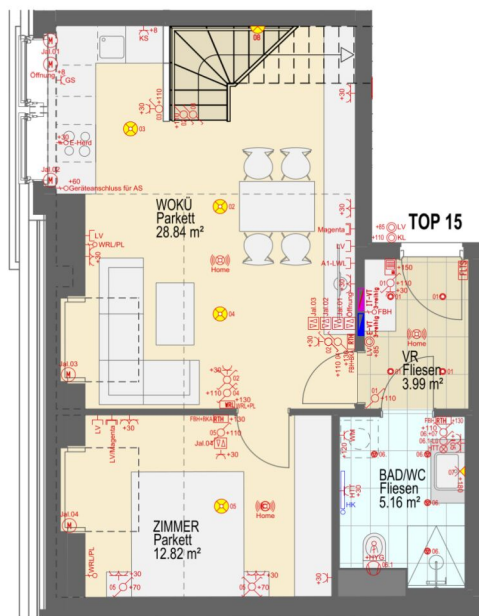
1. Dachgeschoss
