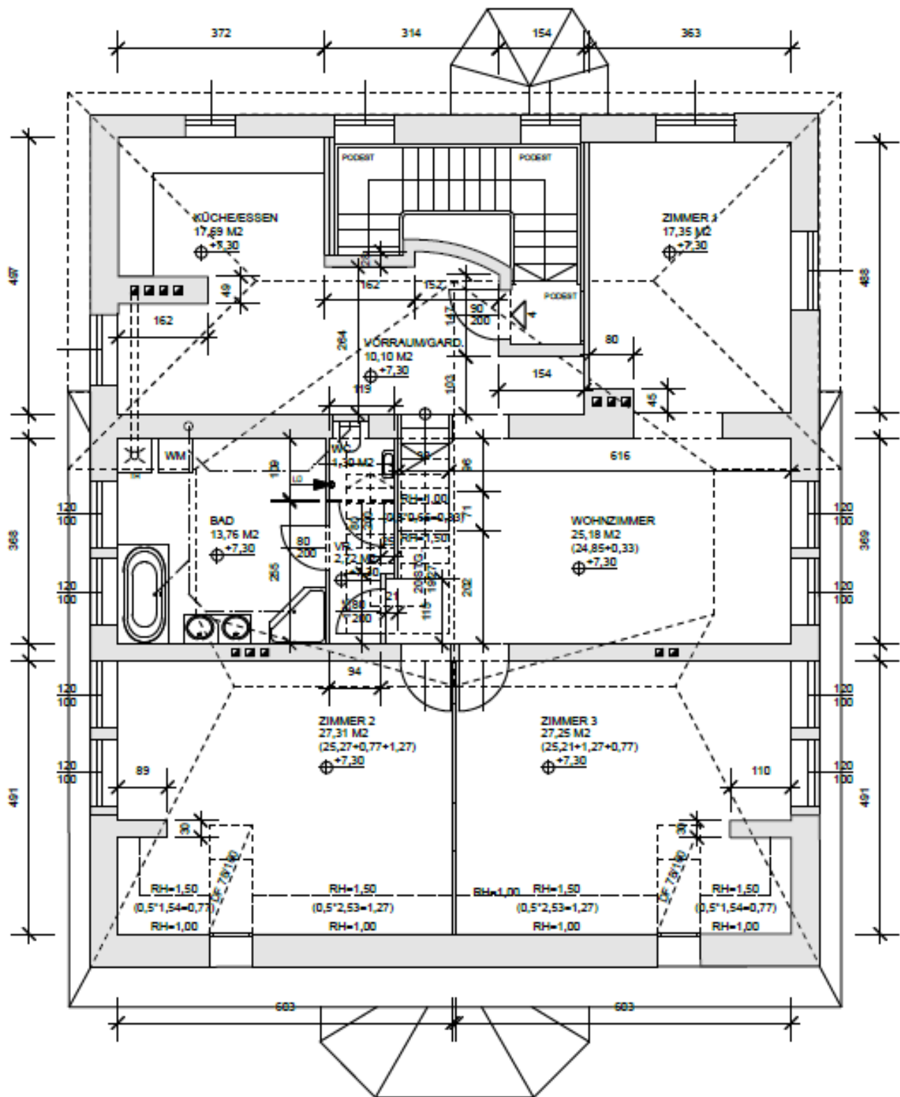
DACHGESCHOSS, M=1:100 TOP 4: 160,34 M 2 (+24,00 M 2 TERRASSE)
