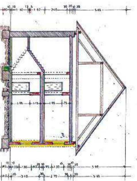
SCHNITT A-B
