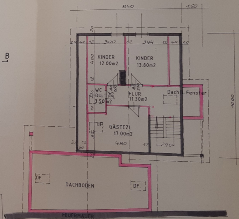
DACHGESCHOSS
