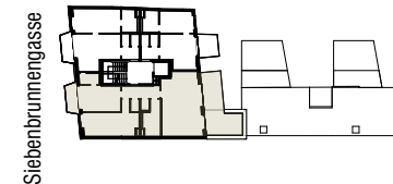
Grundriss 4. Obergeschoss
