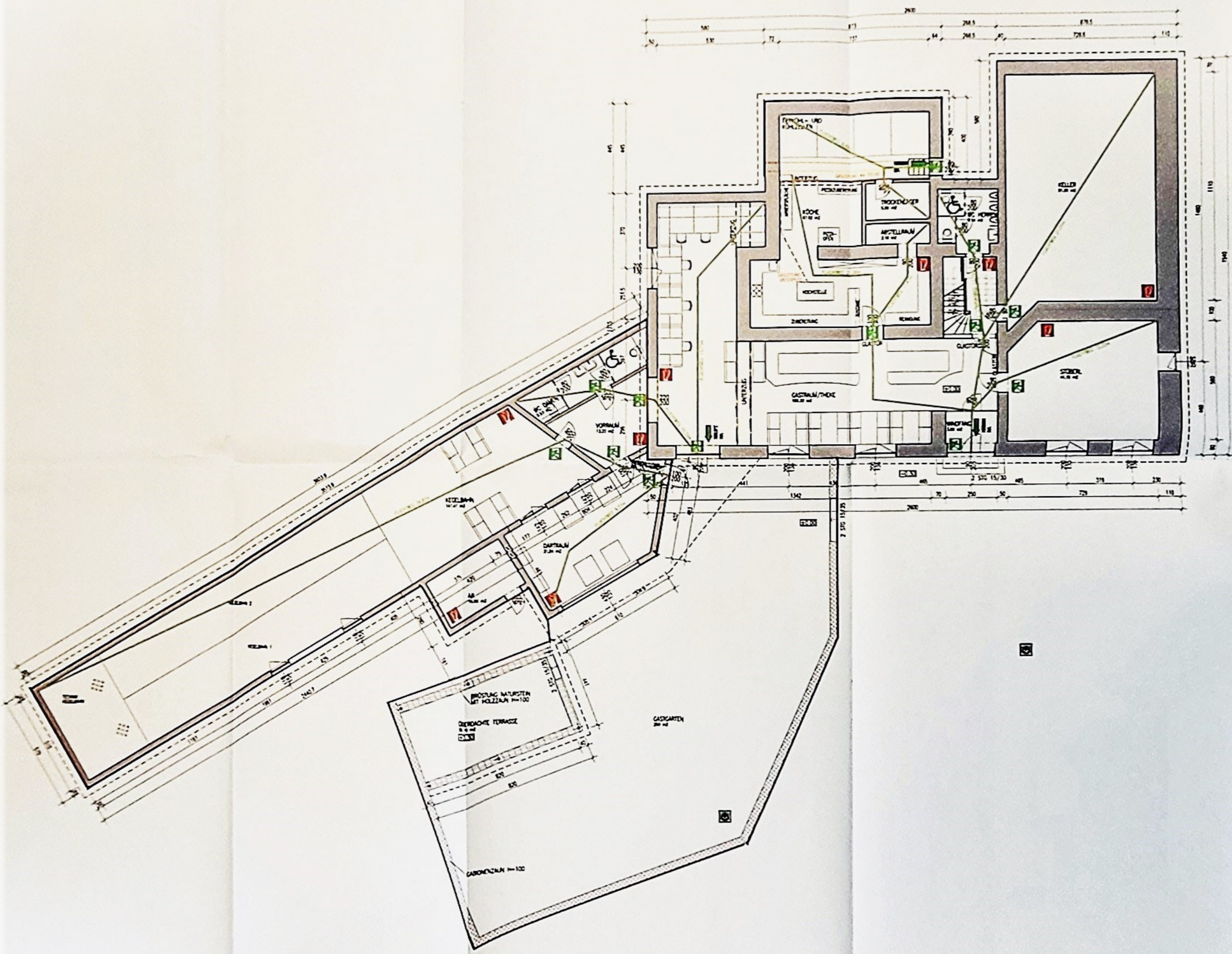
ERDGESCHOSS
