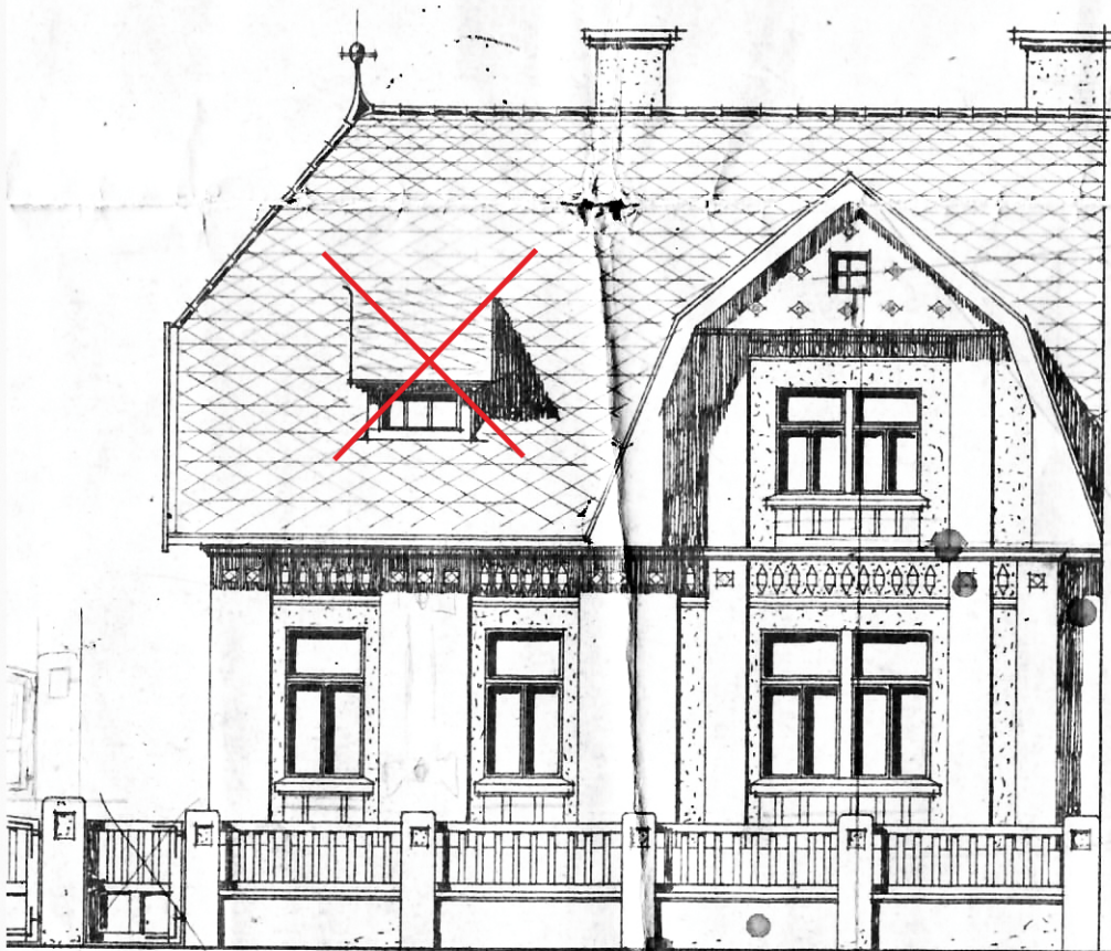
Vorderansicht.
