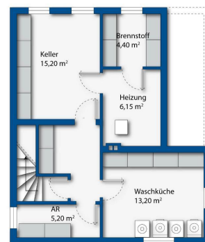
Grundriss KG
