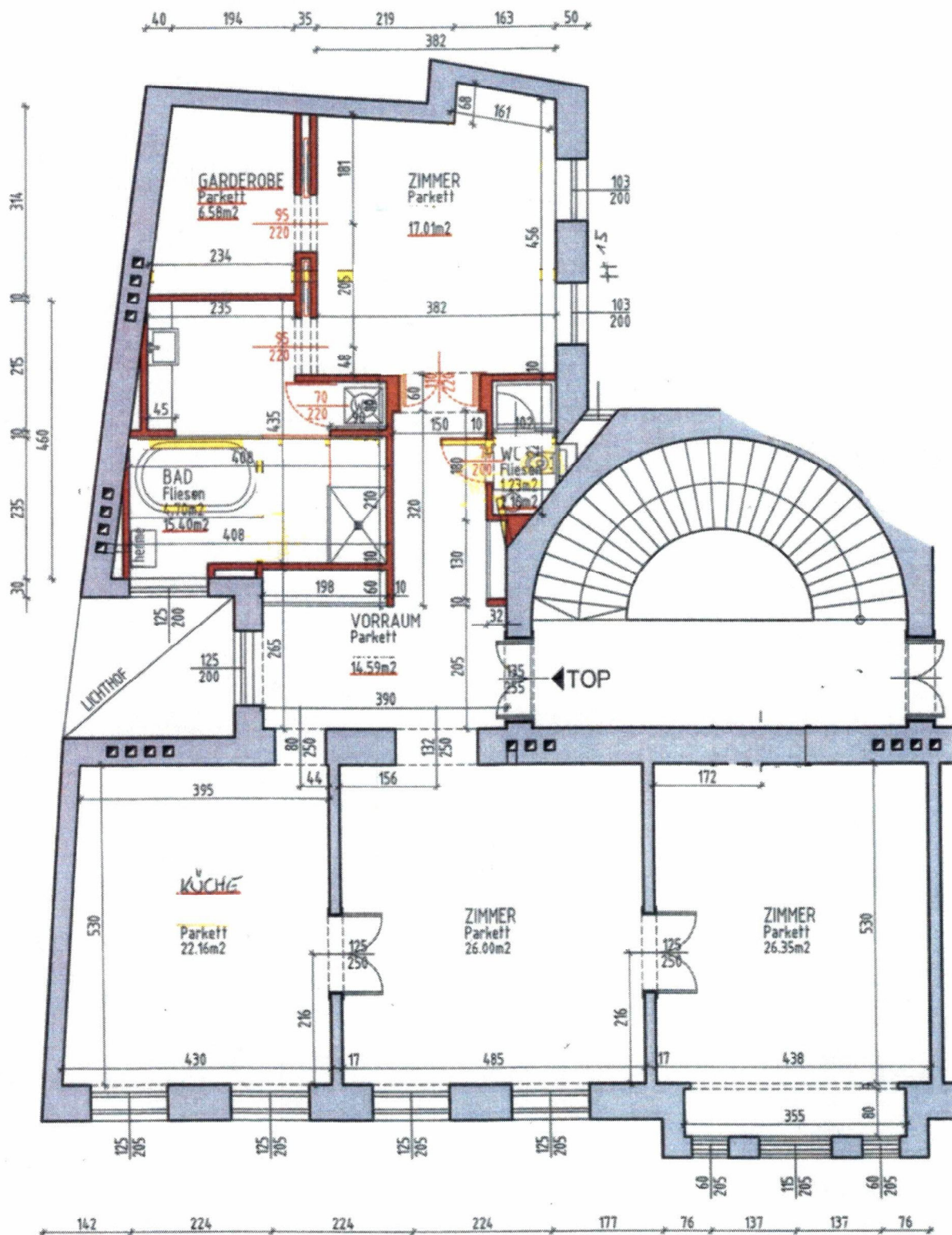
GRUNDRISS
