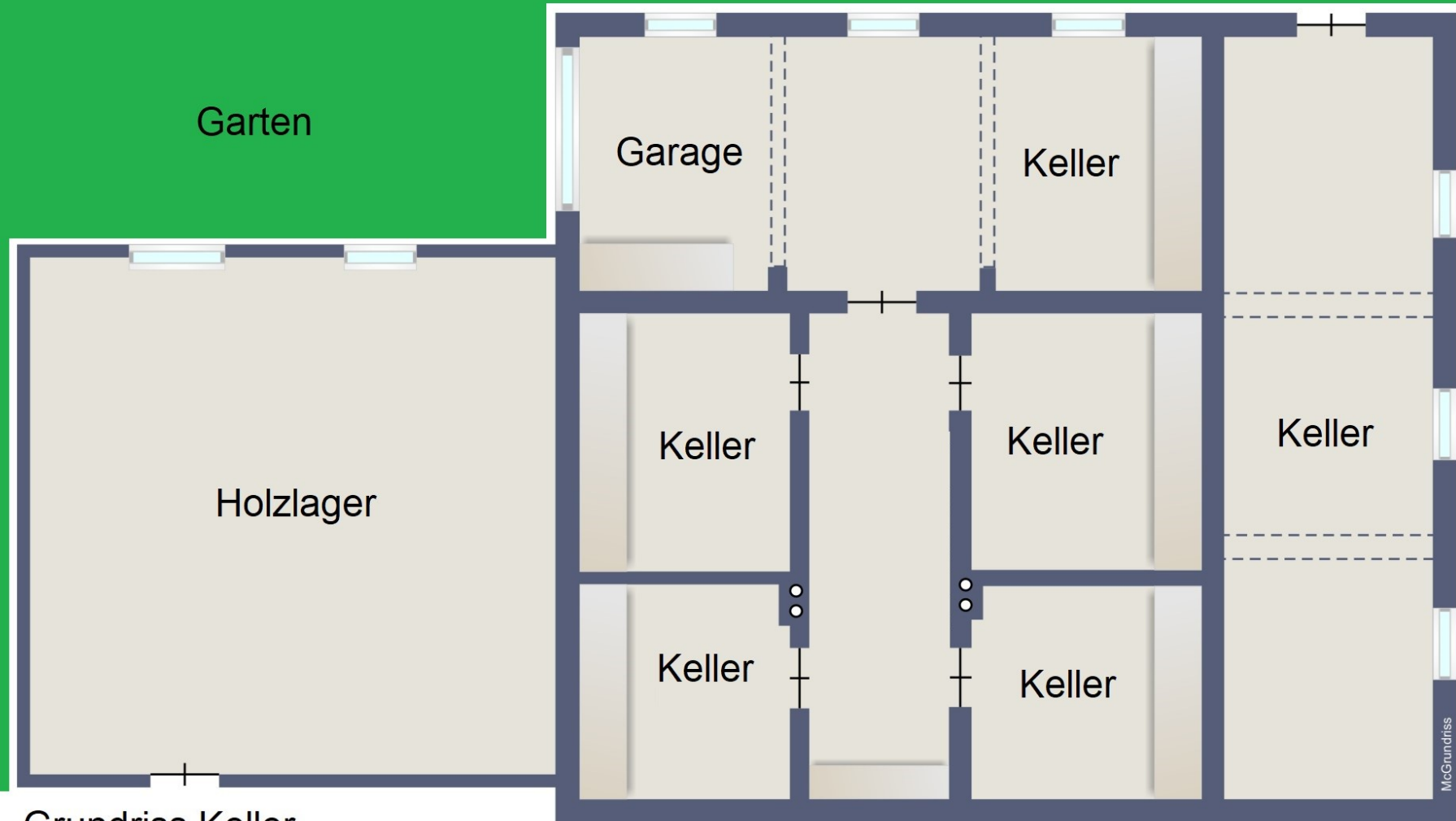
Grundriss Keller
