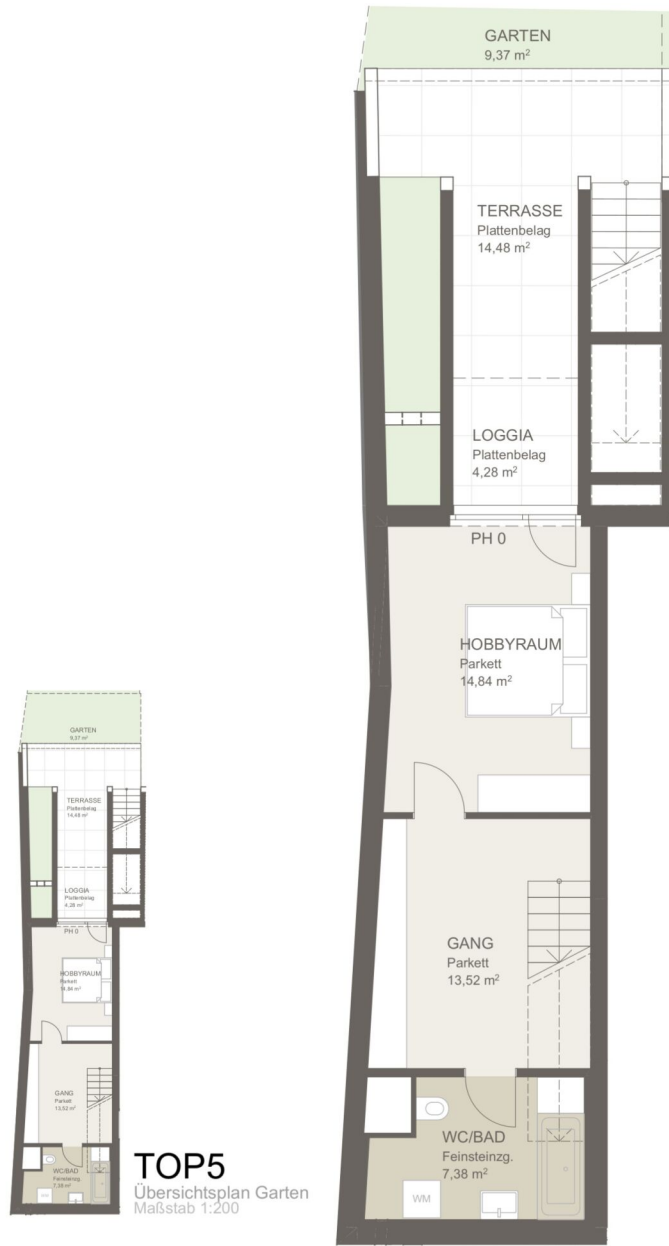
Untergeschoß
