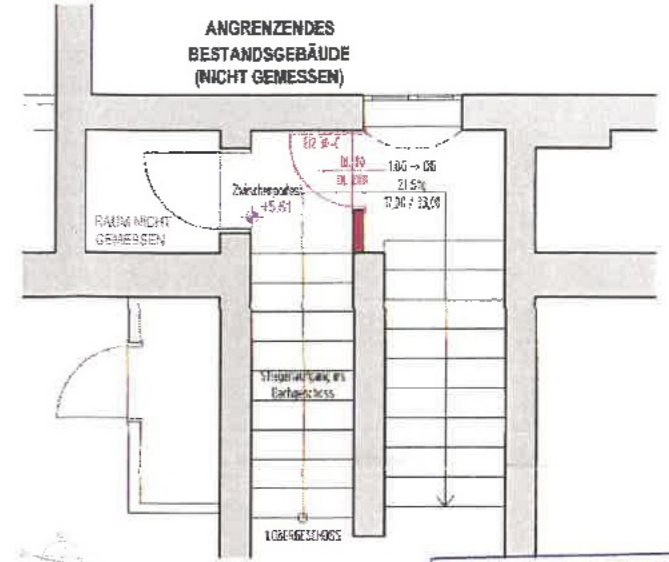
STIEGENAUFANG 1.OG - DG M 1:50
