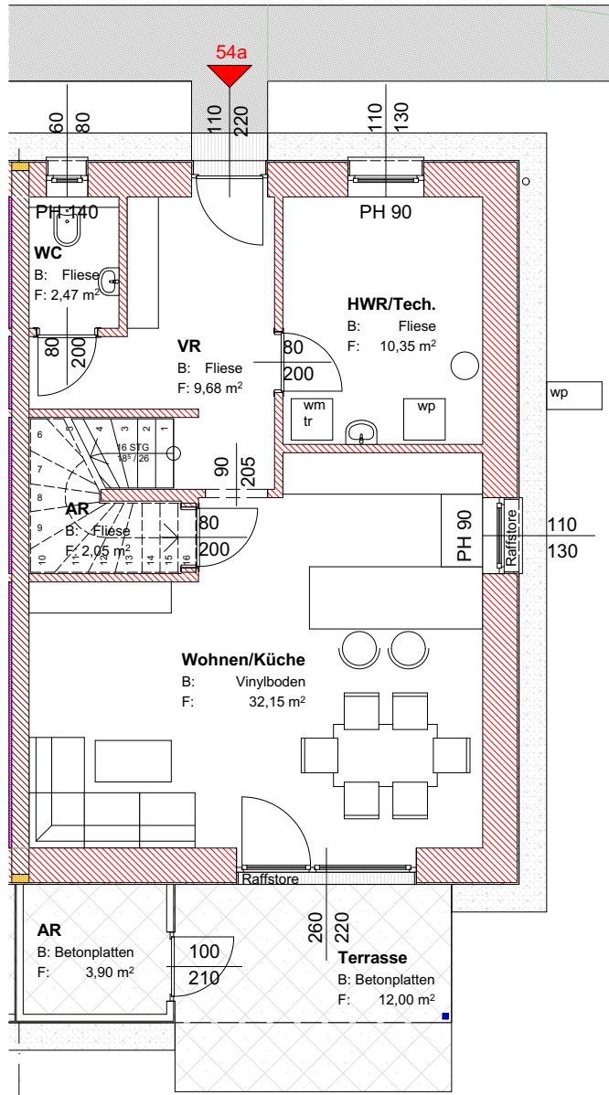
0. Erdgeschoss 1:100
