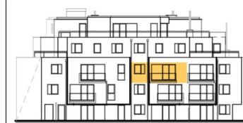
ANSICHT STIEGE 4
