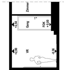
Schnitt
