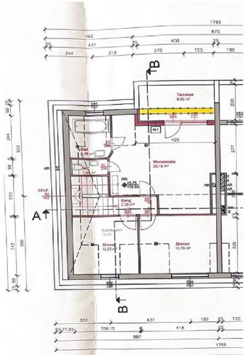
ENTWURF DACHGESCHOSSGRUNDRISS
