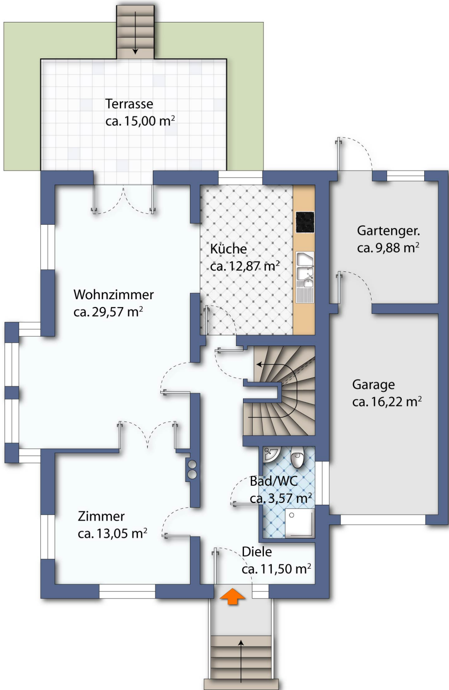
Erdgeschoss: Grundriss-Skizze ohne Gewähr.
