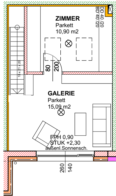
1. OBERGESCHOSS
