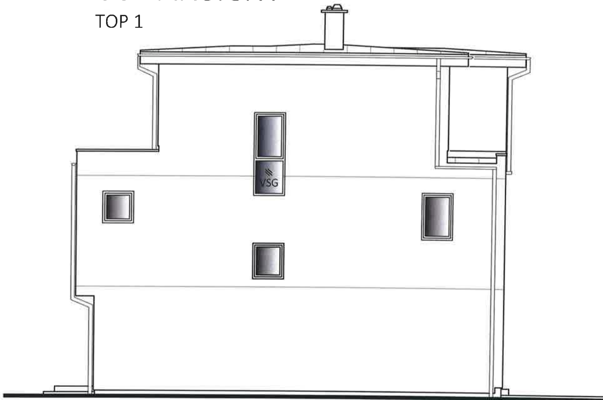
WEST ANSICHT TOP 1
