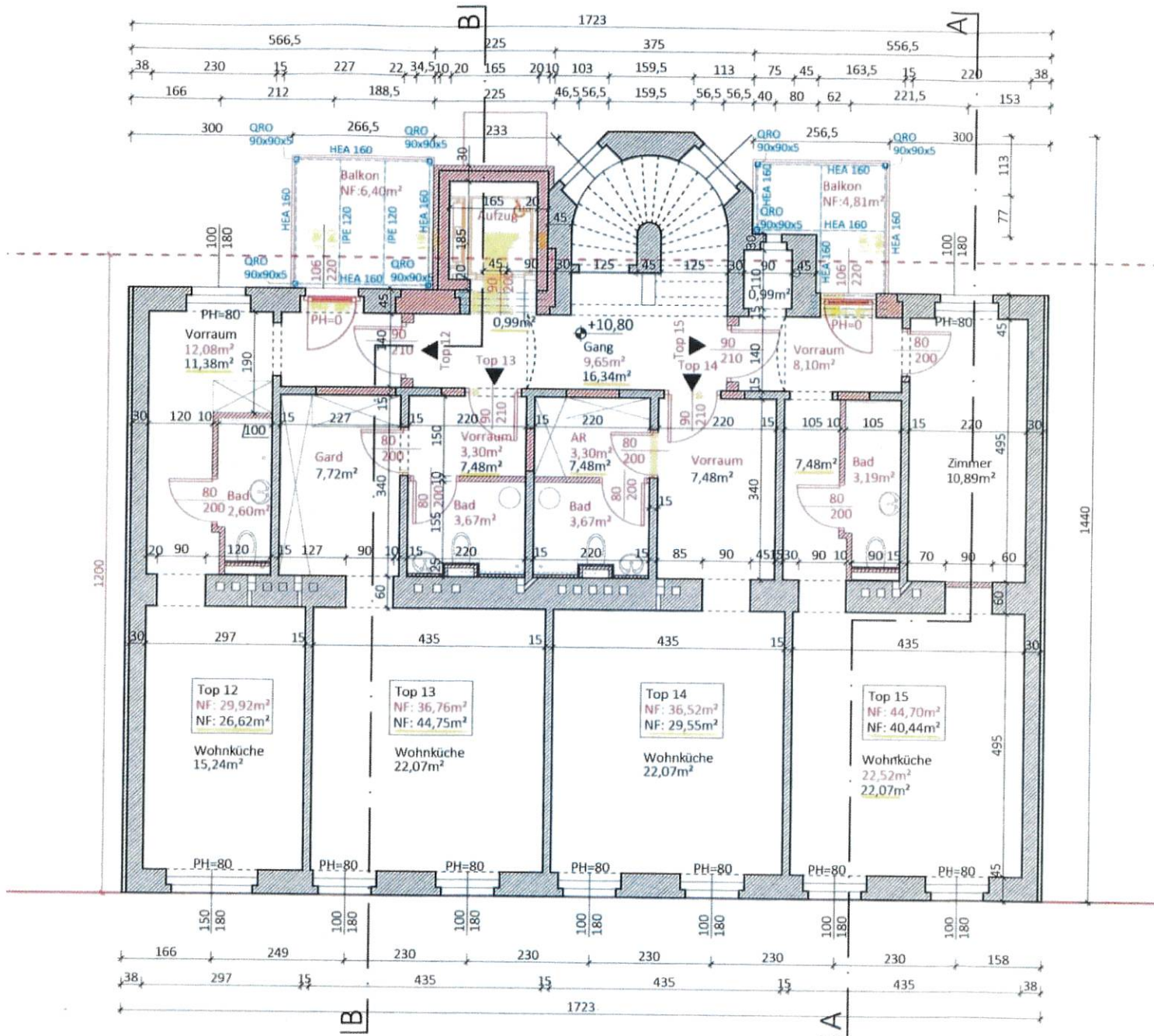
Grundriss 3.Obergeschoss
