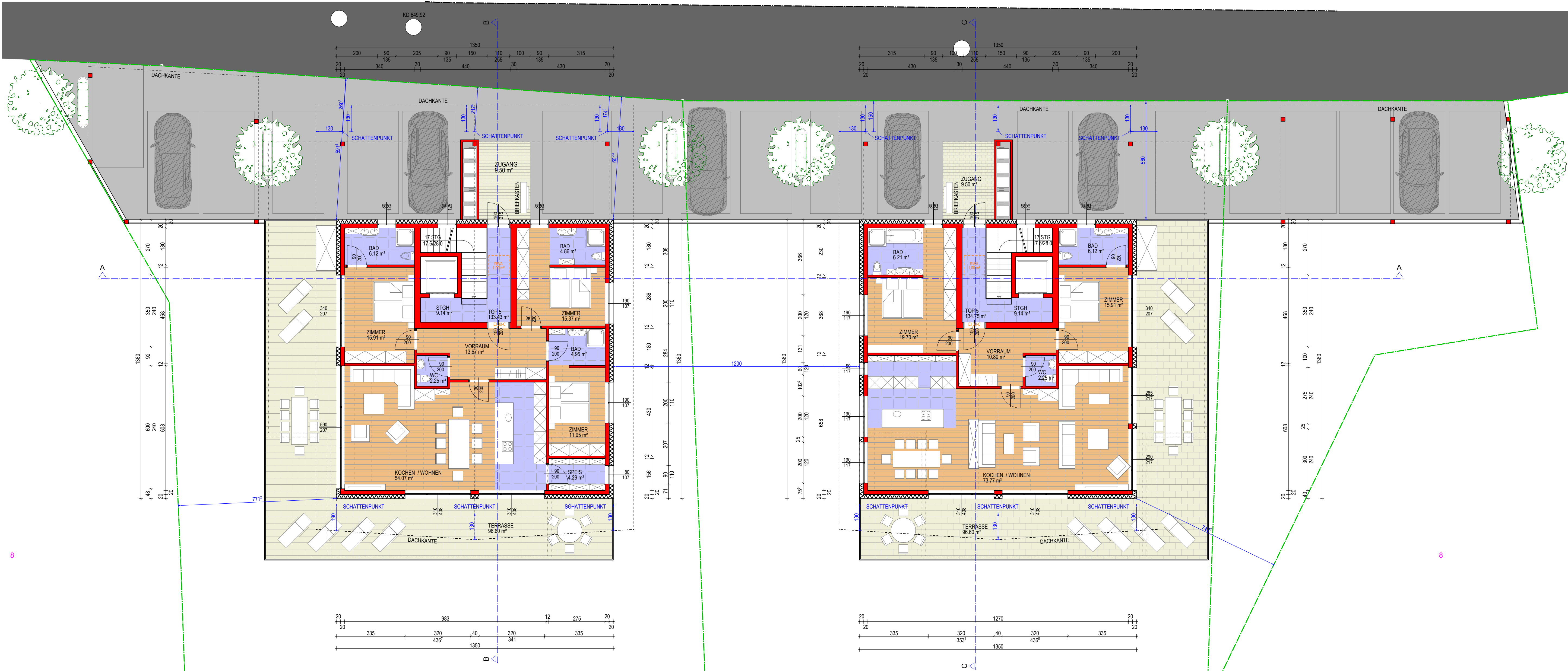
OBERGESCHOSS
