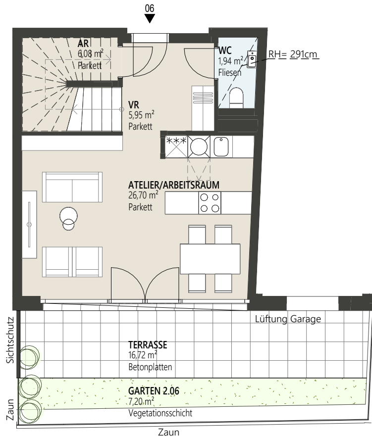
ERDGESCHOSS
