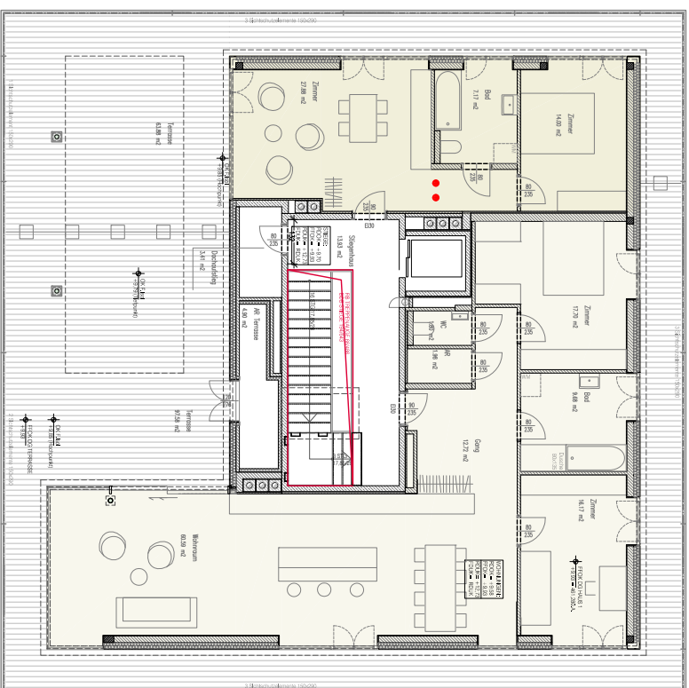
TOP 132 89.04 m 2 DACHGESCHOSS TOP 131 120.64 m 2 STAND 31.03.11
