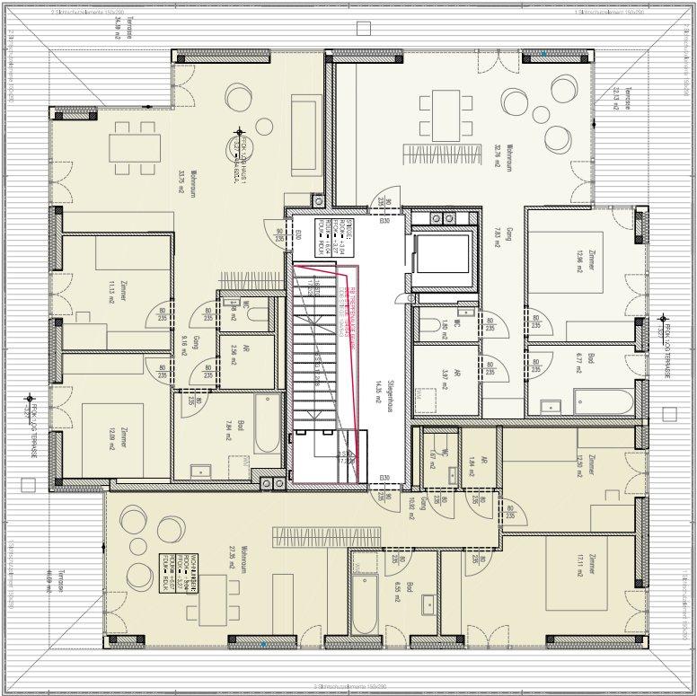
1. OBERGESCHOSS TOP 113 78.03 m 2 TOP 111 77.93 m 2
