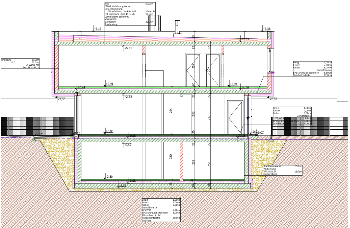
SCHNITT A-A
