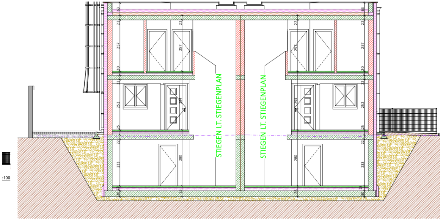
D SCHNITT D-D
