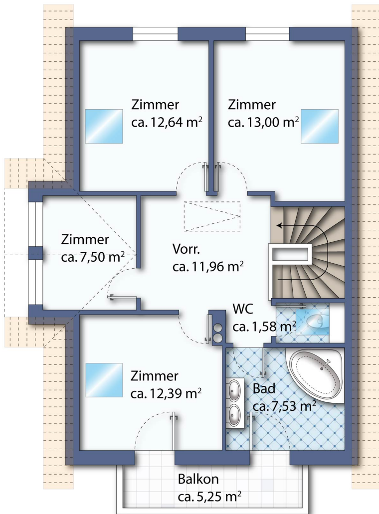
Dachgeschoss: Grundriss-Skizze ohne Gewähr.
