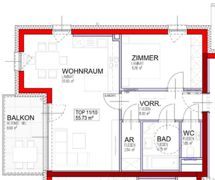
GRUNDRISS 1. OBERGESCHOSS
