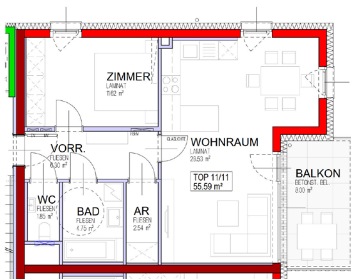
GRUNDRISS 2. OBERGESCHOSS
