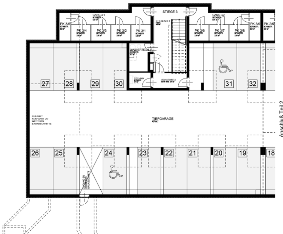
ÜBERSICHT KELLERGESCHOSS TEIL 3
