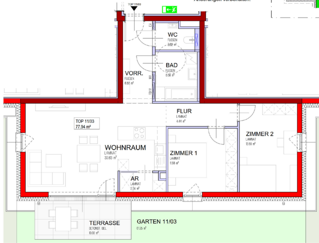
GRUNDRISS ERDGESCHOSS 0 1 2 3 4 5m
