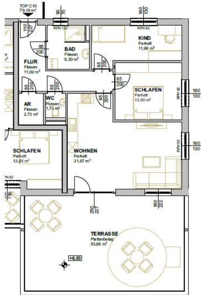
2. OBERGESCHOSS
