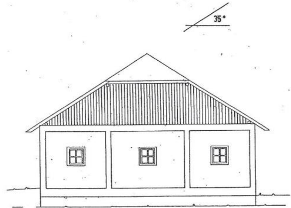
STADL SÜDANSICHT
